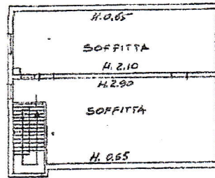
PIANTA PIANO SOFFITTA (2°) H medio m. 1.58
